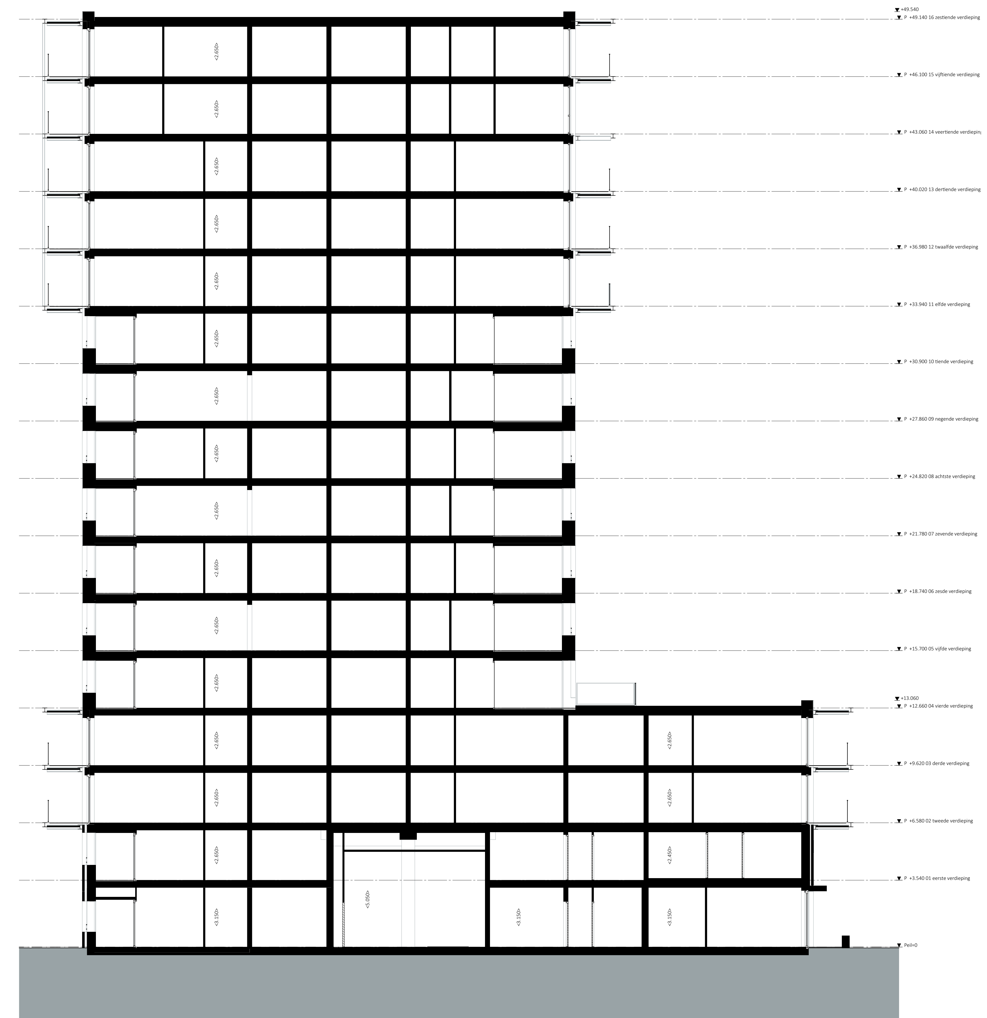
Doorsnede C-C
