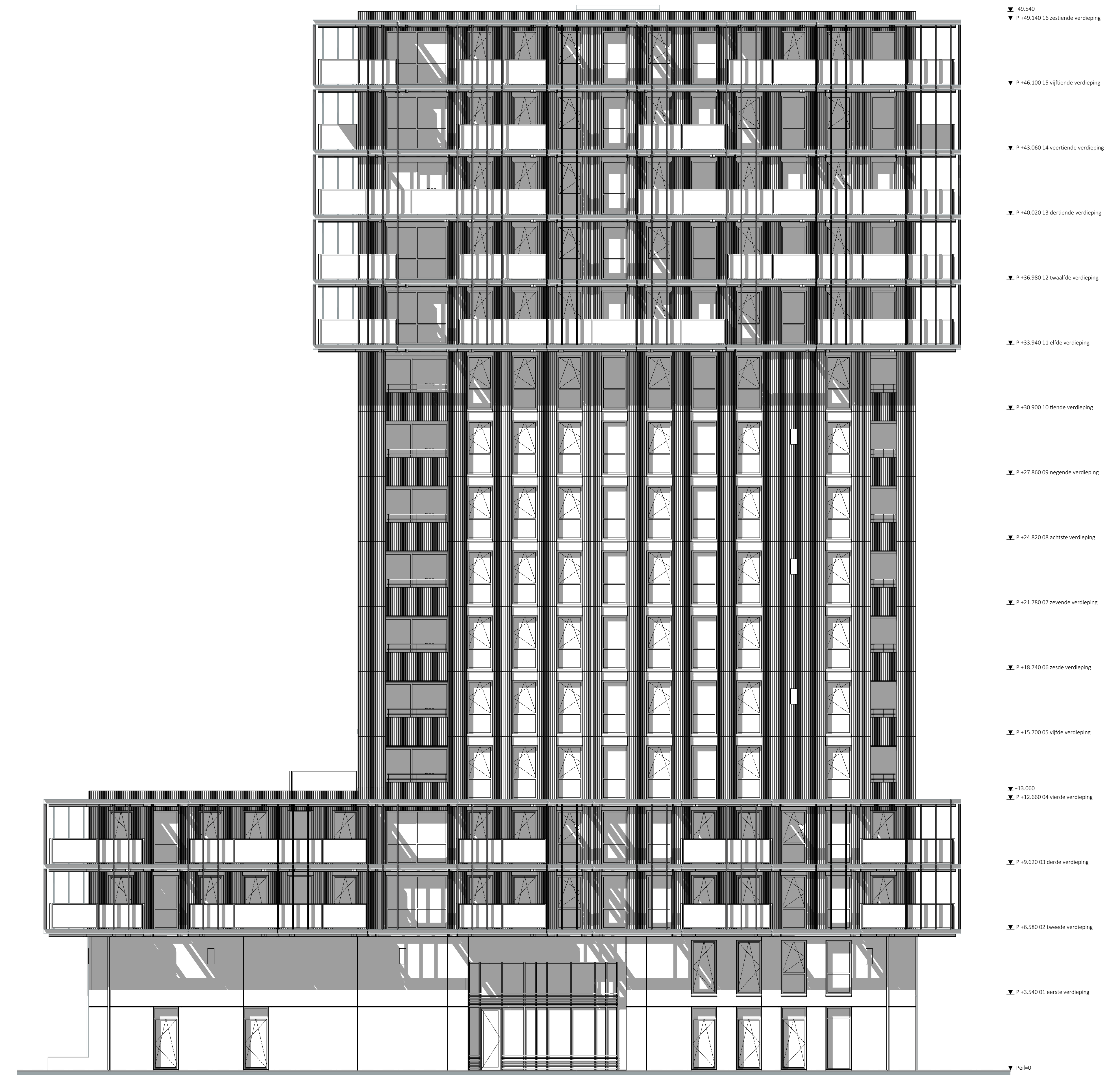
Noordgevel
