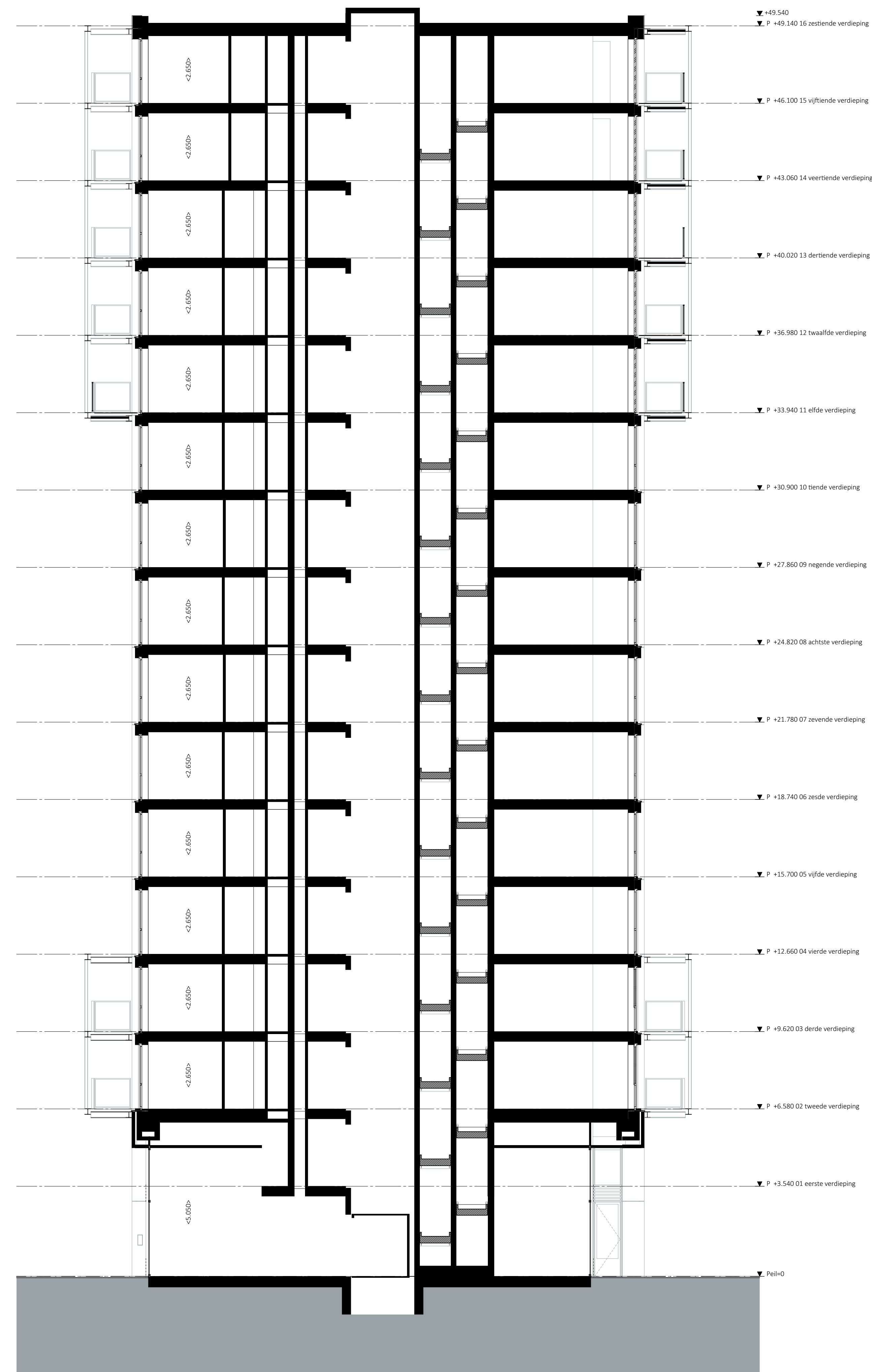
Doorsnede B-B
