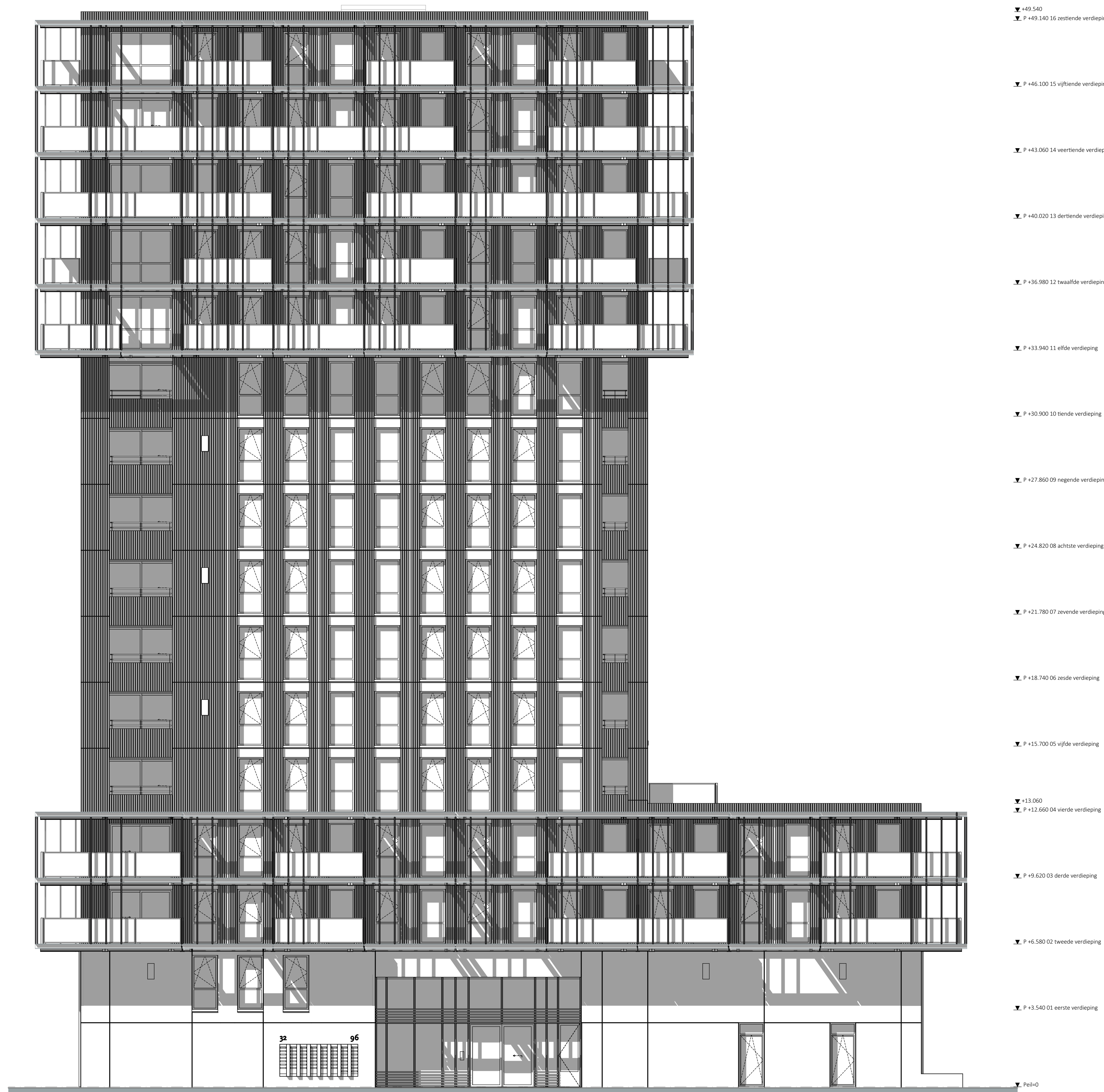
Zuidgevel
