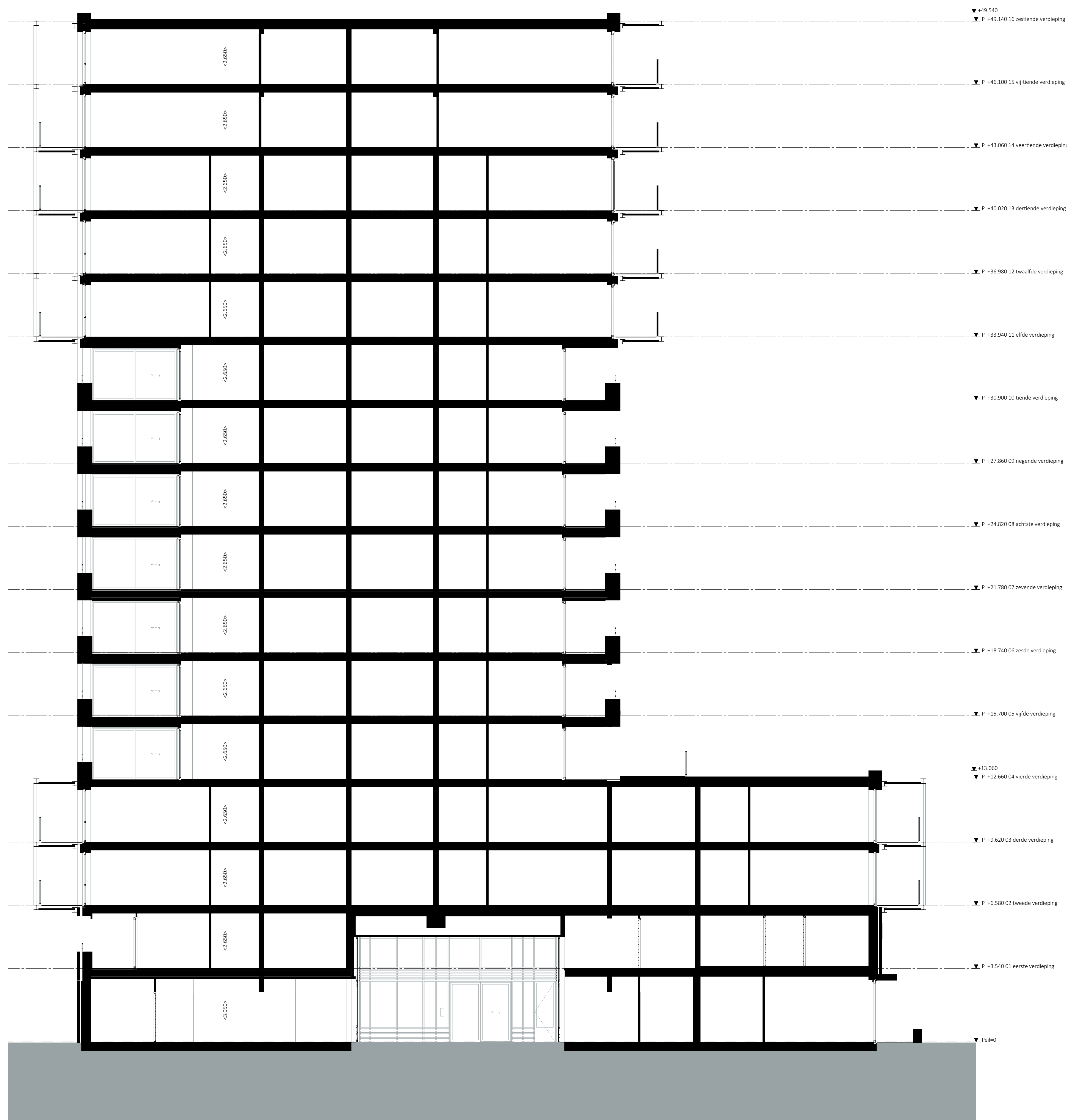
Doorsnede A-A
