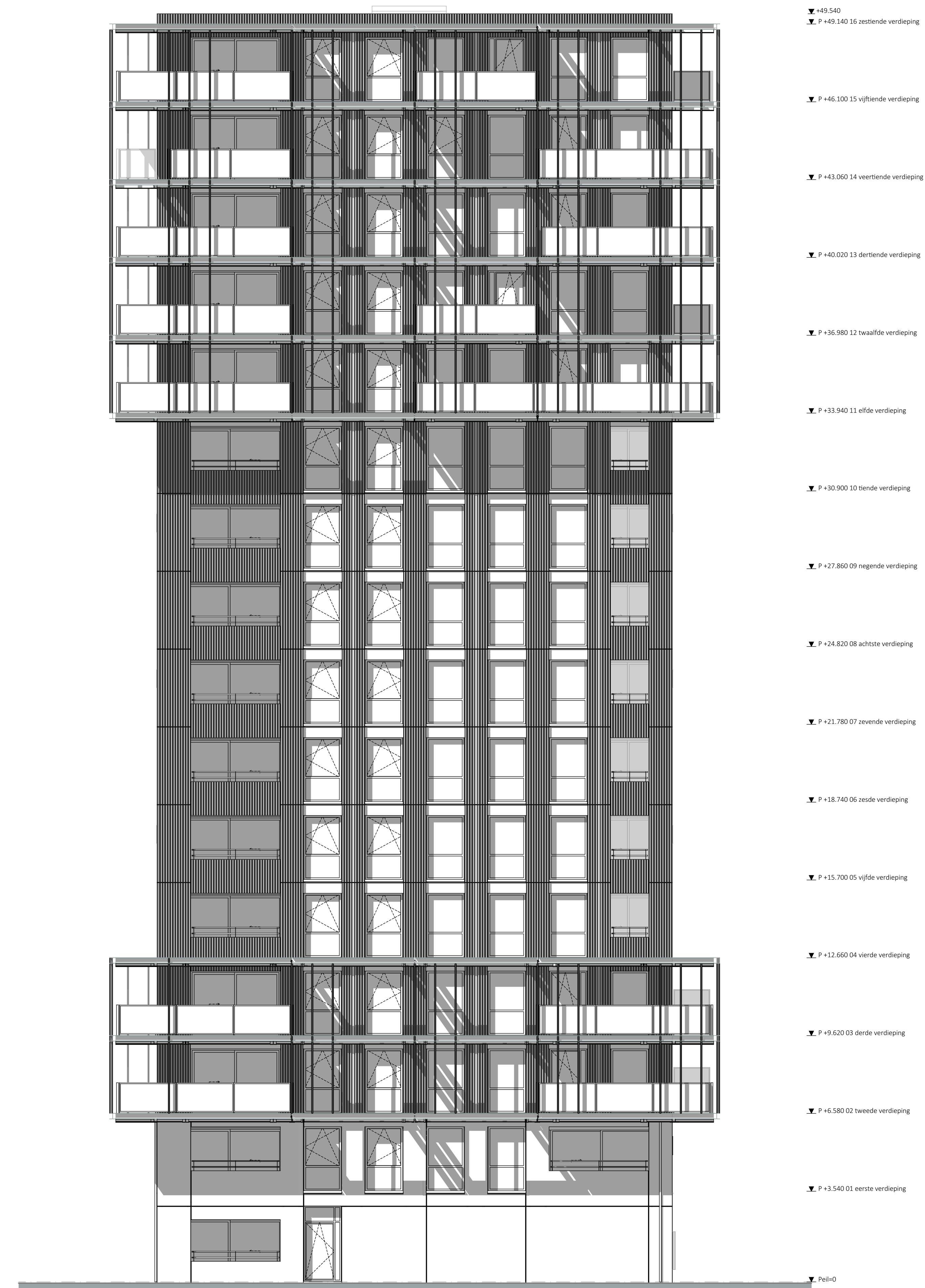
Westgevel
