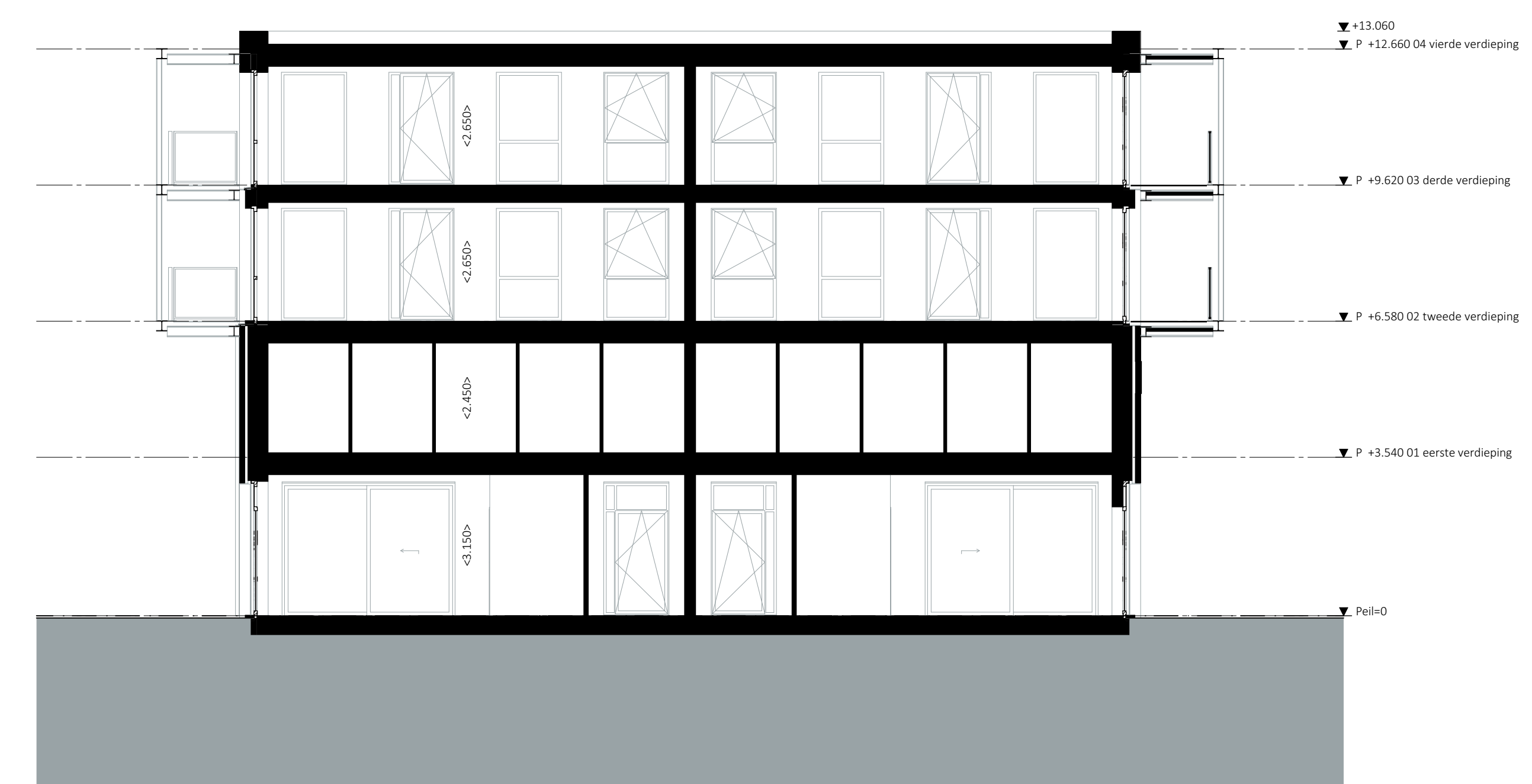
Doorsnede D-D
